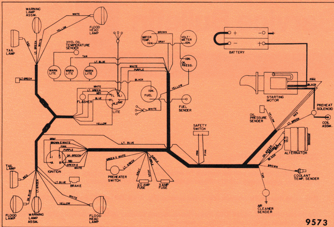
Fig. 1. Voltmeter Wiring Diagram
