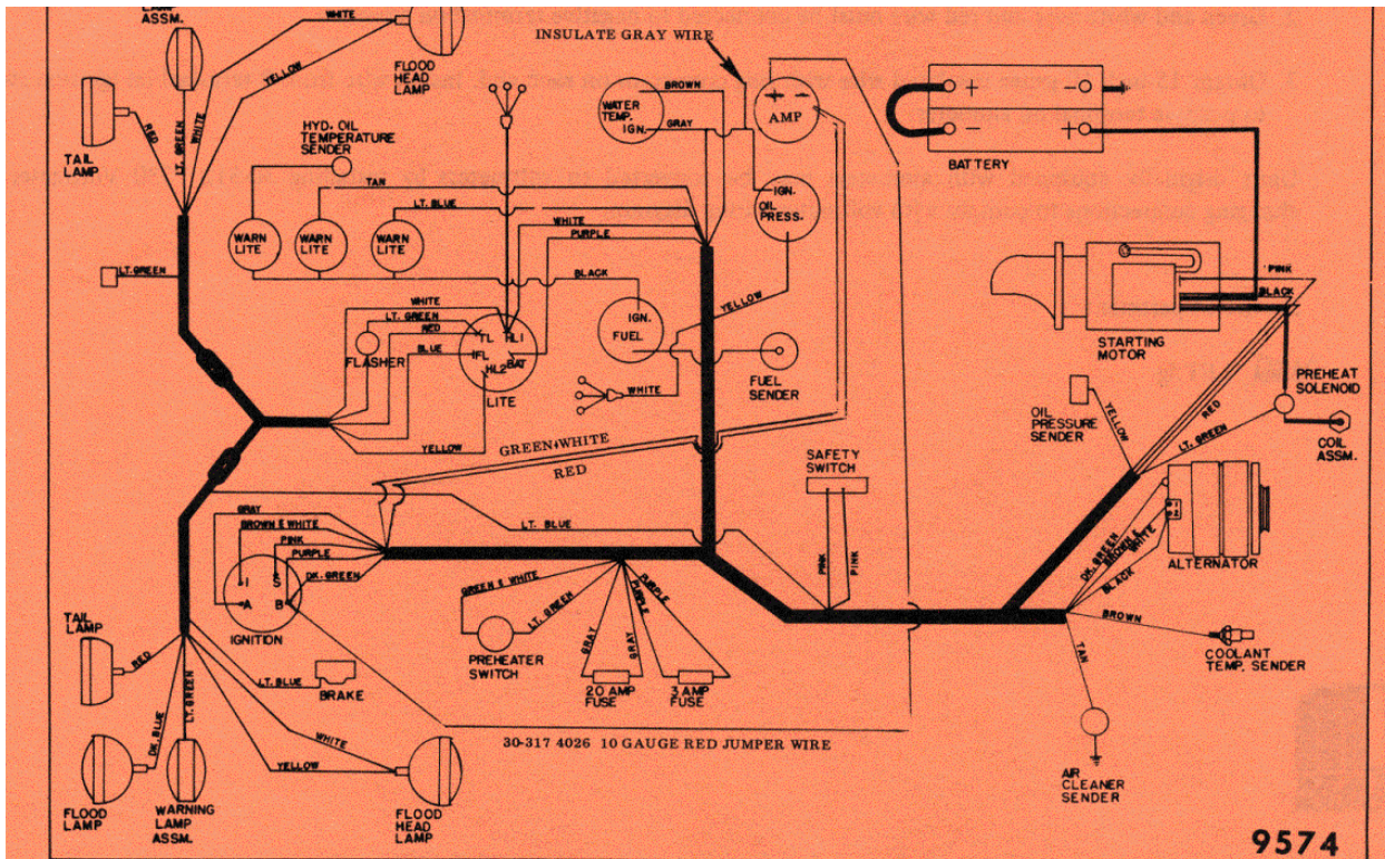
Fig. 2. Ammeter Wiring Diagram
